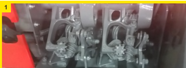
Vista posteriore della macchina al lavoro Rear view of the machine at work
